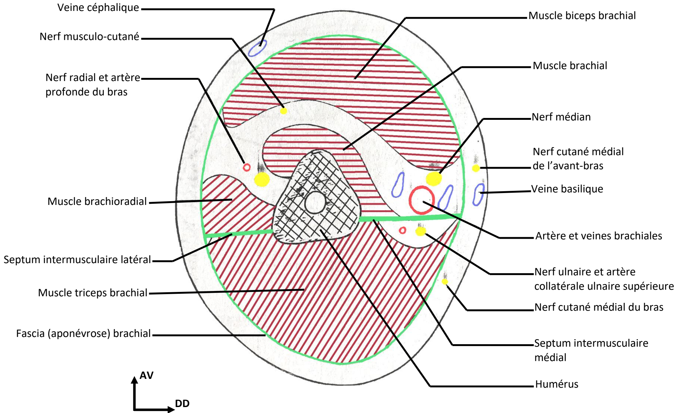
Coupe transversale du bras droit passant à l'union du tiers moyen et du tiers inférieur
